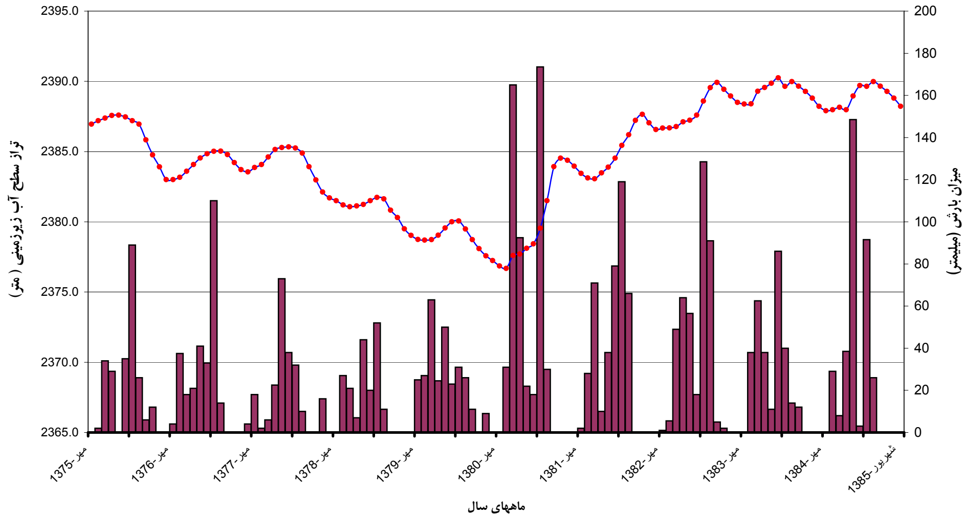
نمودار شماره (۱-۳): هیدروگراف معرف آبخوان ابرفتی محدوده مطالعاتی چهل خانه همراه با بارش ماهانه همزمان در ایستگاه بارانسنجی میرآباد
